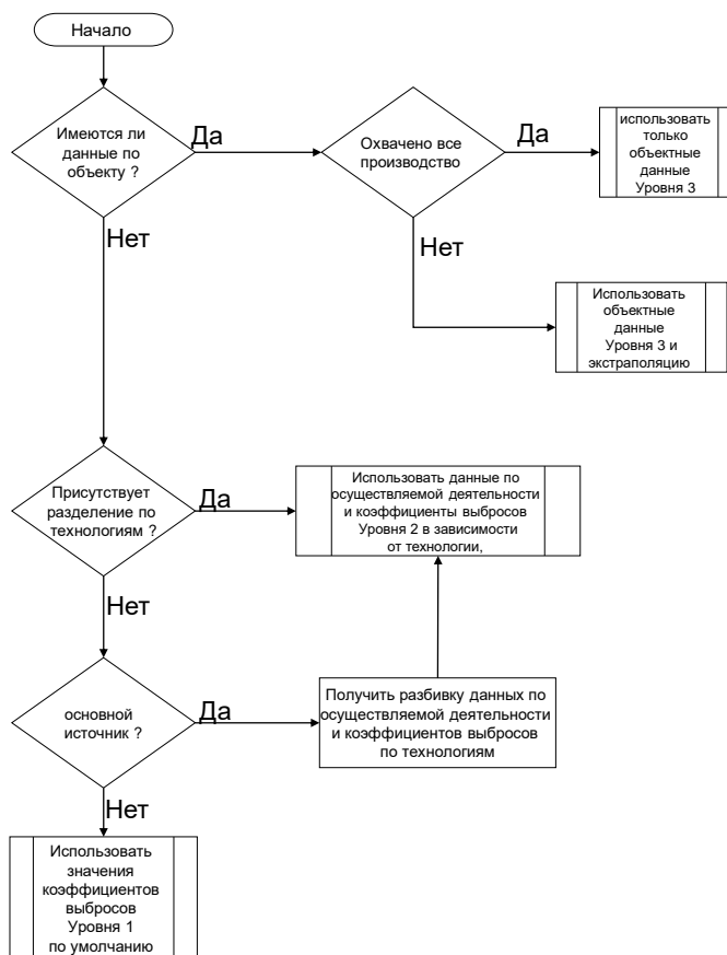
Рисунок 3-1 Дерево решений для категории источника 5.С.1.в.iii Сжигание медицинских отходов
