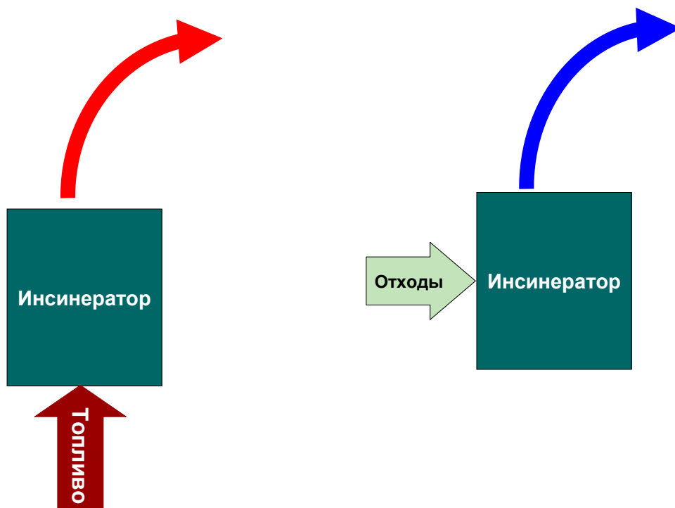
Рисунок 2-1 Схема процесса для категории источника 5.С.1.в.iii Сжигание медицинских отходов; слева показана схема с использованием вторичного тепла; справа – без использования вторичного тепла
