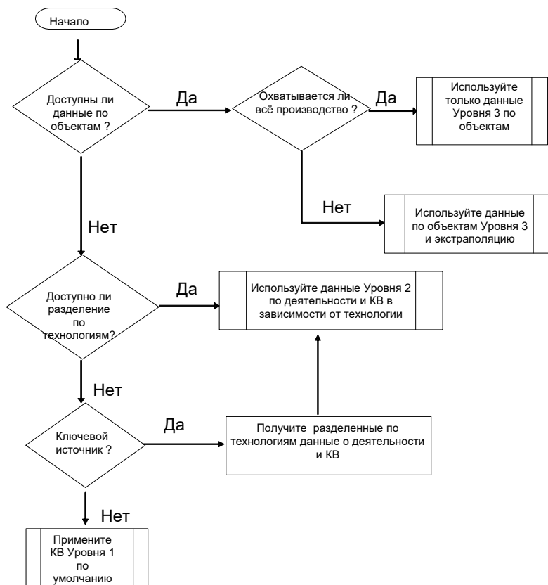
Рисунок 3-1 Схема принятия решений для категории 2.A.1 Производство цемента
