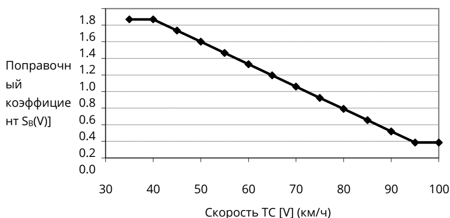
Рисунок 3-3 Поправочный коэффициент на скорость для выбросов частиц износа тормозов
