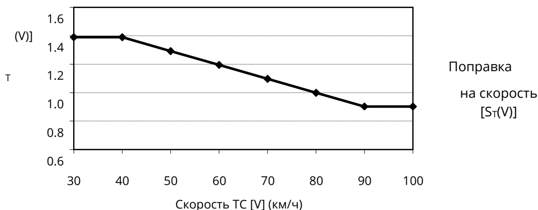
Рисунок 3-2 Поправочный коэффициент на скорость для выбросов частиц износа покрышек
