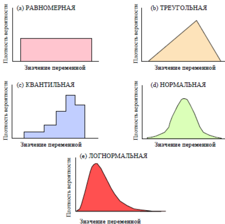
Рисунок А-1 Примеры некоторых широко используемых моделей плотности распределения вероятностей (напр. по Фрею и Рубину, 1991 г.)
