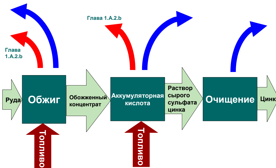
Рисунок 2.2 Схема процесса для категории источника 2.С.6 Производство цинка, процесс производства цинка электрохимическим способом
