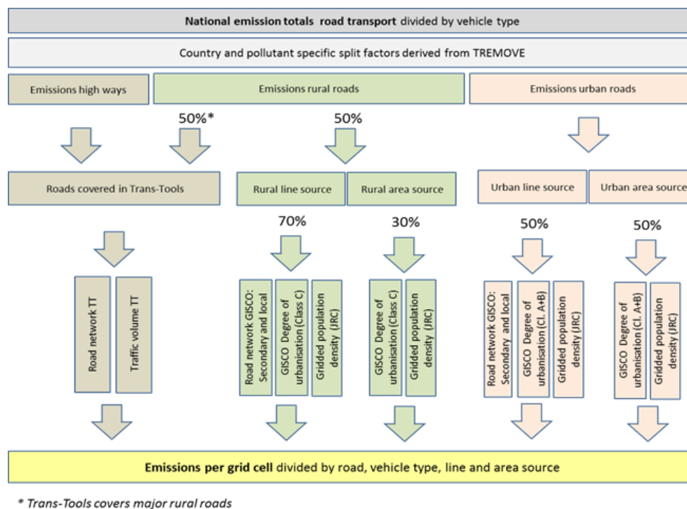
Рисунок 3-3 Обзор применяемой методологии для пространственного распределения дорожного транспорта, Theloke et al. (2009).
