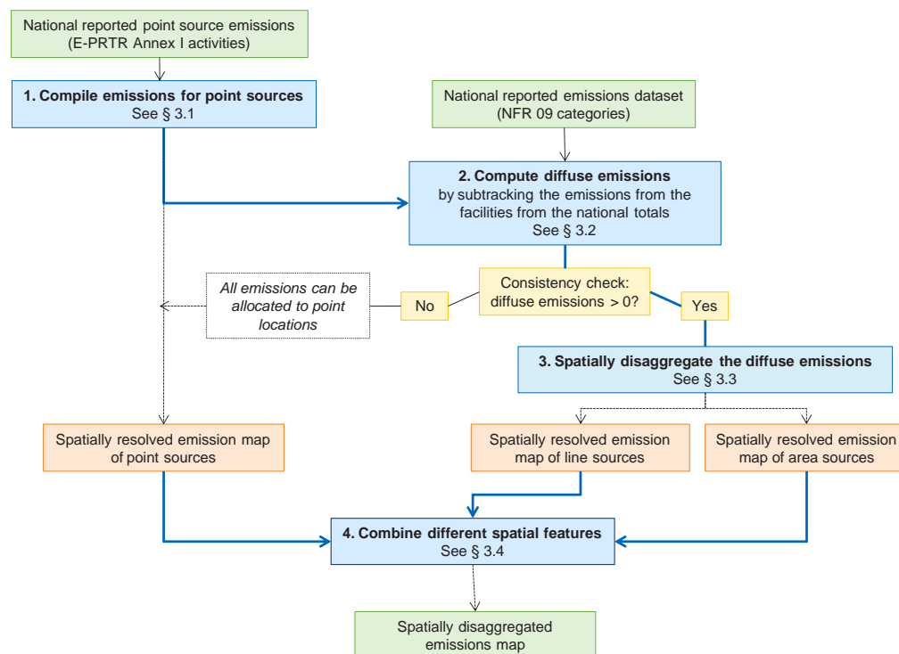
Рисунок 3-1 Общий подход к составлению инвентаризации пространственных выбросов
