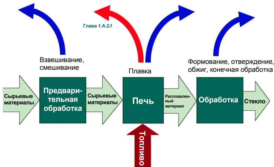
Рисунок 2.1 Технологическая схема 2.А.7.d Добыча других полезных ископаемых, применяемых для производства стекла
