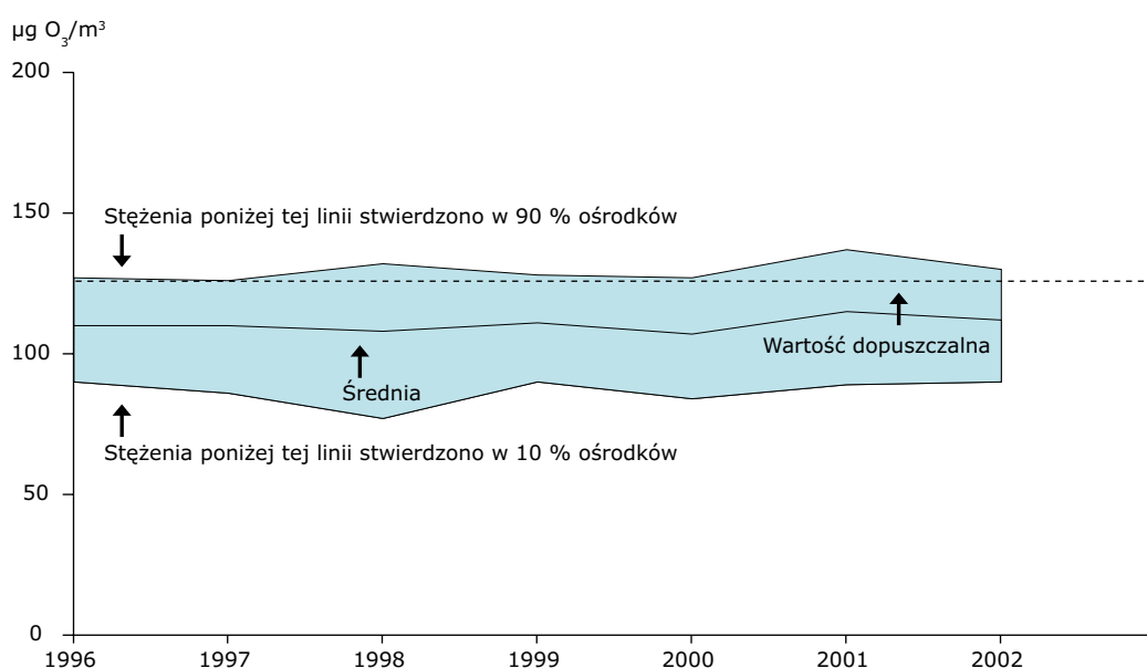
Rycina 4 Maksymalne stężenie ozonu (26. maksymalna dobową średnia z 8 godz.) obserwowane w miejskich stacjach monitorujących stężenia tła (kraje członkowskie EEA), lata 1996–2002
