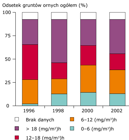
Rycina 2 Narażenie upraw na działanie ozonu (narażenie wyrażone jako AOT40 w (\text{mg}/\text{m}^3)\text{h} w krajach członkowskich EEA, lata 1996–2002 (2) )
