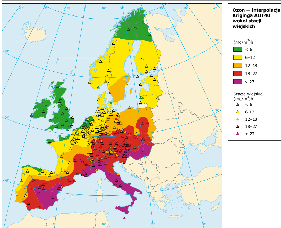
Mapa 1 Narazienie na AOT40 powyżej wartości docelowych w odniesieniu do roślinności wokół wiejskich stacji monitorujących stężenie ozonu (kraje członkowskie EEA, 2002 r.)
