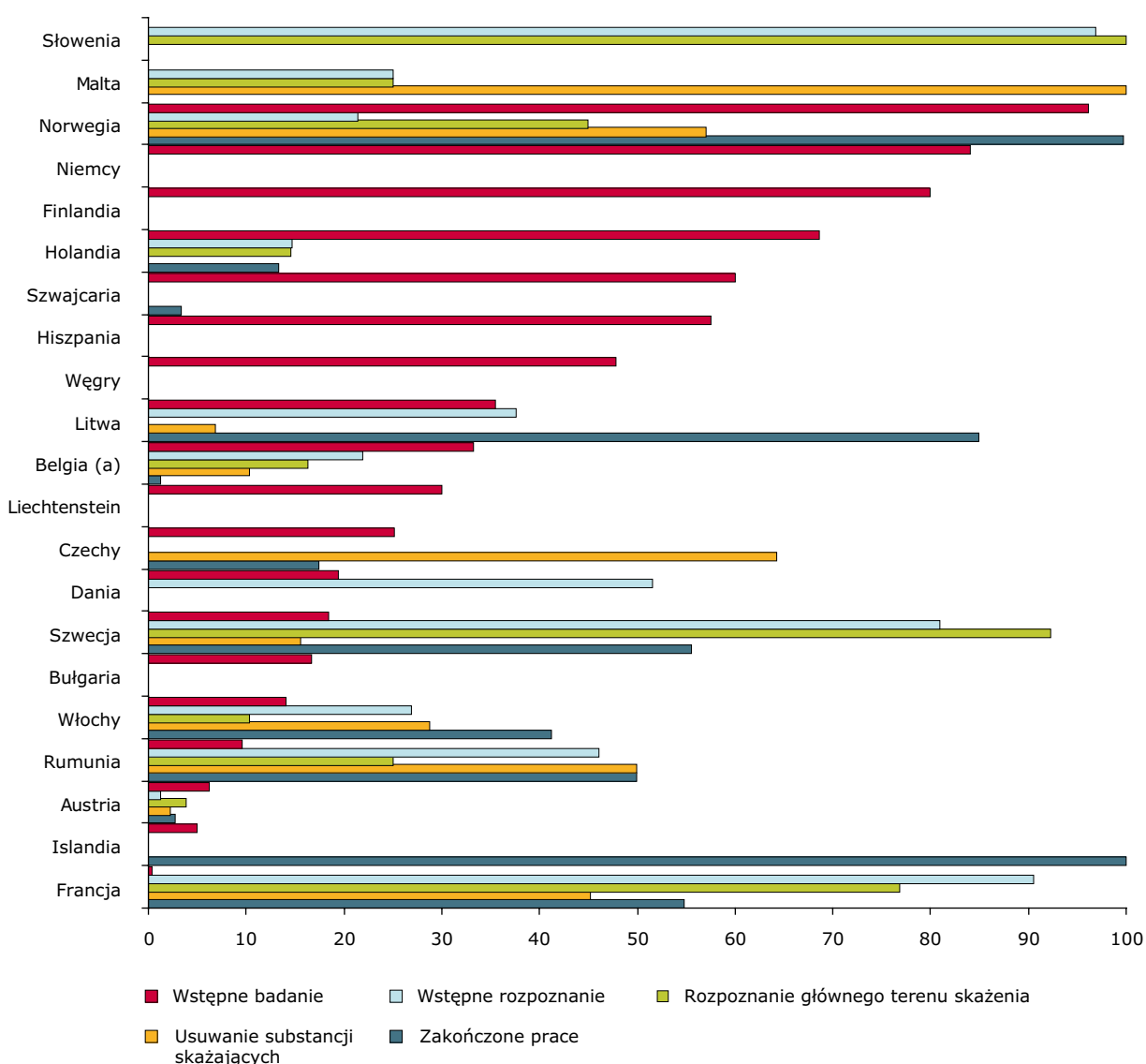
Rycina 1 Przegląd postępów prac z zakresu ograniczania i usuwania substancji skażających glebę wg krajów
