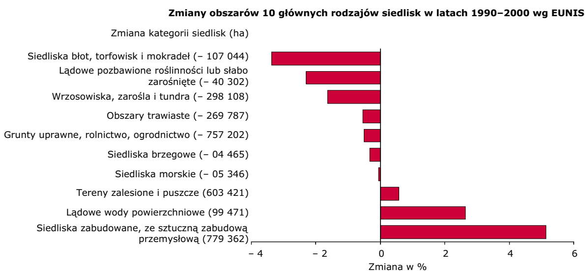
Rycina 2 Zmiany zagospodarowania gruntów w latach 1990–2000 wyrażone jako % poziomu z 1990 r., zgrupowane w kategorii poziomu 1 siedlisk wg EUNIS
