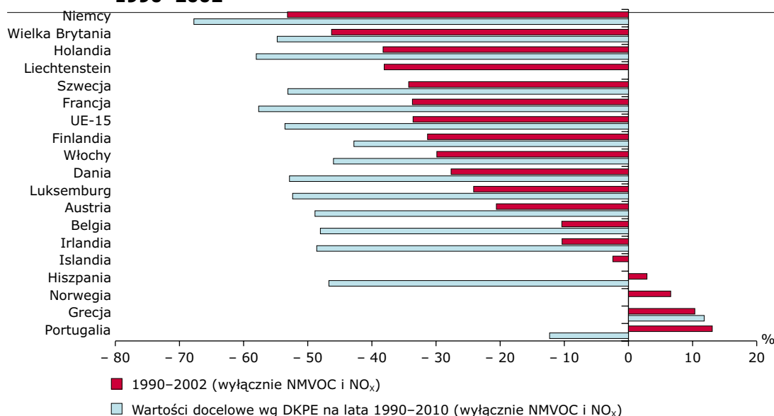
Rycina 3 Zmiany emisji prekursorów ozonu (EFTA-3 i UE-15) w porównaniu do wartości docelowych na rok 2010 określonych w DKPE (wyłącznie UE-15), lata 1990–2002
