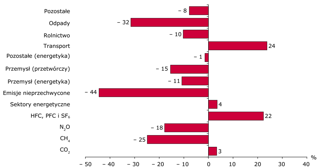
Rycina 4 Zmiany emisji gazów cieplarnianych według sektorów i według rodzajów gazów na terenie UE-15 w latach 1990–2003
