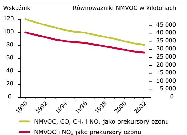
Rycina 1 Trendy emisji prekursorów ozonu (równoważniki NMVOC w kilotonach) w krajach członkowskich EEA, lata 1990–2002
